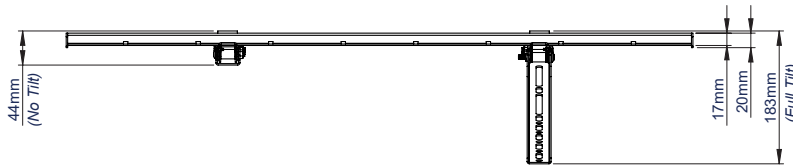
VISTA SUPERIOR
