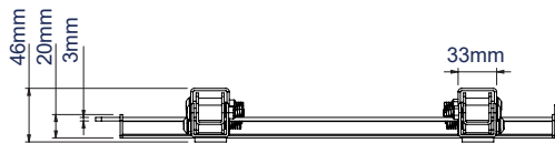
VISTA SUPERIOR
