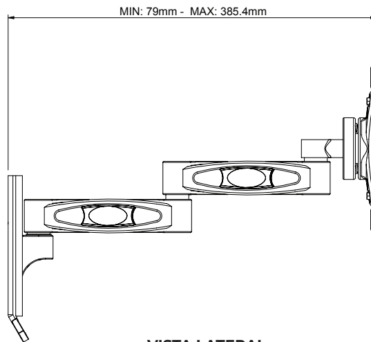
VISTA LATERAL CON EL BRAZO EXTENDIDO
