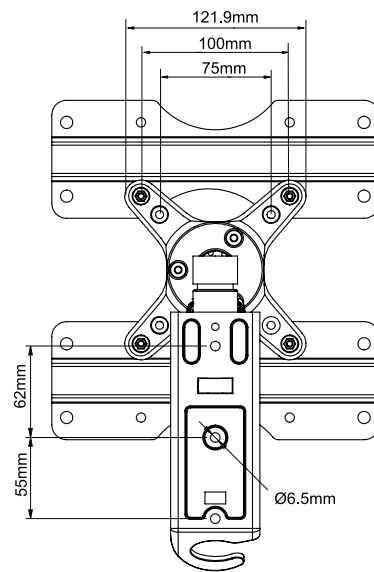
VISTA TRASERA
