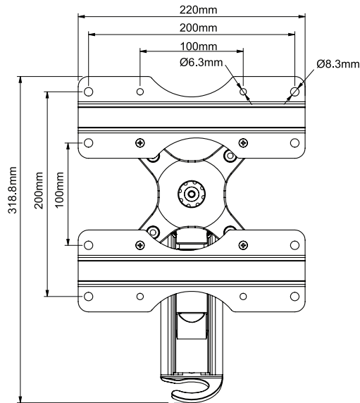
VISTA FRONTAL EXTENSIÓN COMPLETA
