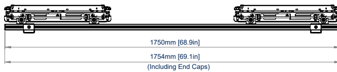
VISTA SUPERIOR
