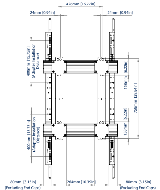
VISTA TRASERA
