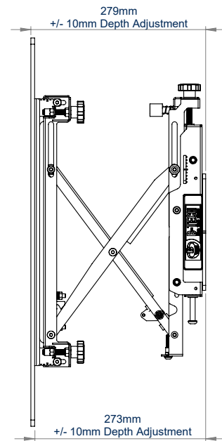
VISTA LATERAL AMPLIADO
