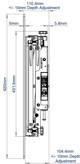
VISTA LATERAL CERRADO
