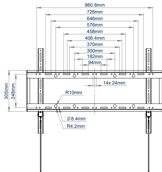
VISTA TRASERA
