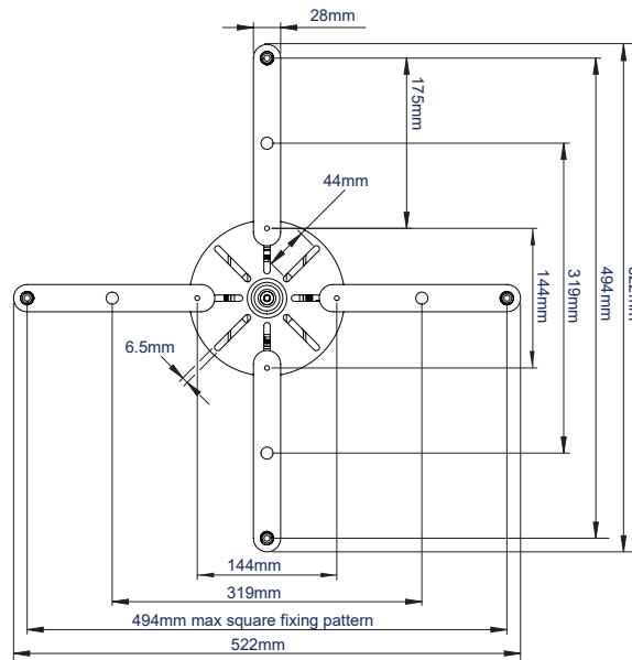
VISTA SUPERIOR CON PATAS EXTENSIBLES GRANDES OPCIONALES
