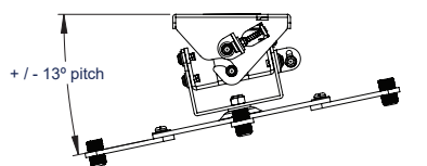
VISTA LATERAL / INCLINACIÓN
