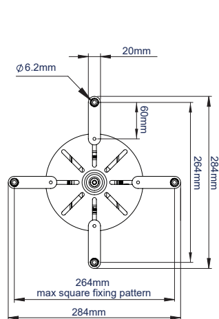
VISTA SUPERIOR CON PATAS DE EXTENSIÓN PEQUEÑAS OPCIONALES
