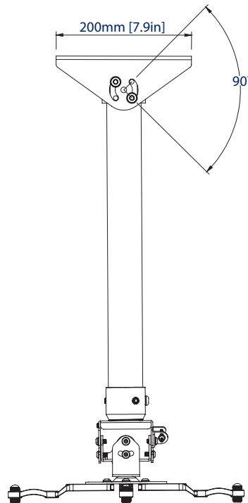
VISTA LATERAL
