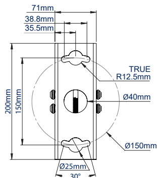
PLACA PARA TECHO O PARED
