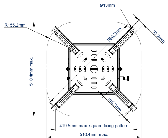
VISTA INFERIOR CON PATAS EXTENSIBLES PEQUEÑAS
