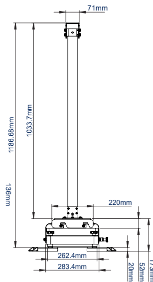
VISTA FRONTAL CON PATAS EXTENSIBLES
