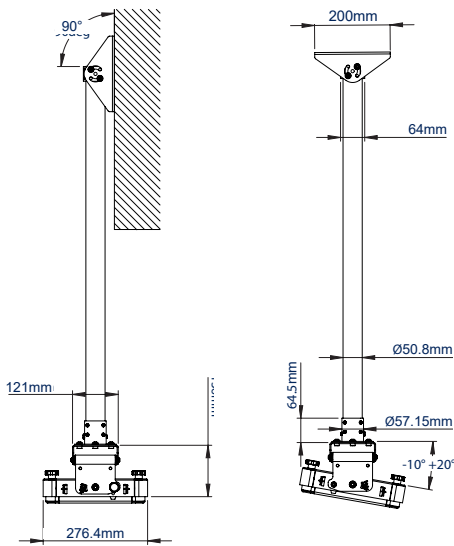
VISTA LATERAL PARA MONTAJE EN PARED
