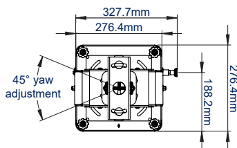
VISTA DESDE ARRIBA
