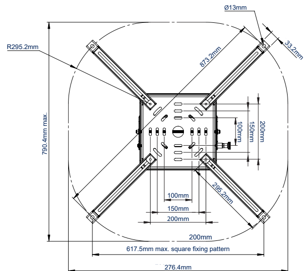
VISTA INFERIOR CON PATAS EXTENSIBLES GRANDES
