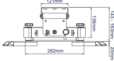
VISTA LATERAL CON PATAS EXTENSIBLES CORTAS INCLUIDAS
