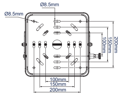
VISTA DESDE ABAJO
