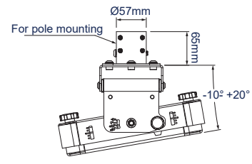
VISTA LATERAL CON ADAPTADOR PARA MÁSTIL INCLUIDO
