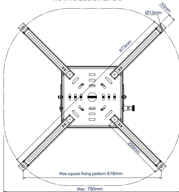
VISTA DESDE ABAJO CON PATAS EXTENSIBLES LARGAS INCLUIDAS
