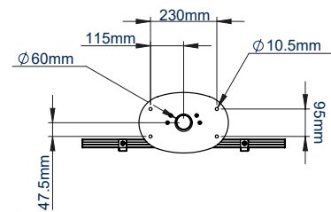
VISTA TRASERA
