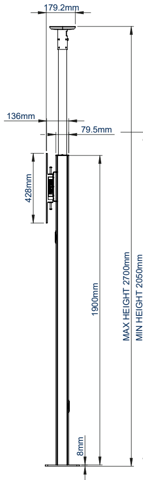
VISTA LATERAL
