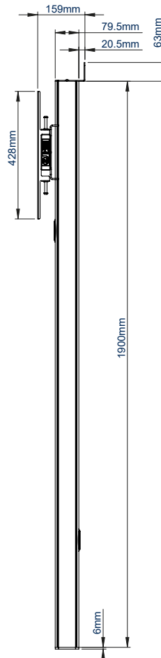
VISTA LATERAL
