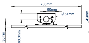
VISTA SUPERIOR
