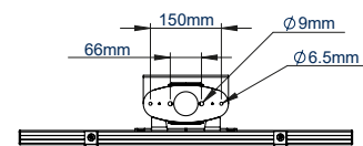
VISTA TRASERA
