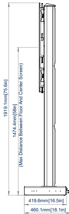
VISTA LATERAL
