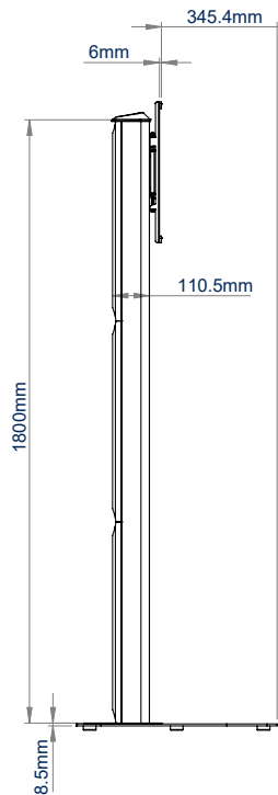
VISTA LATERAL
