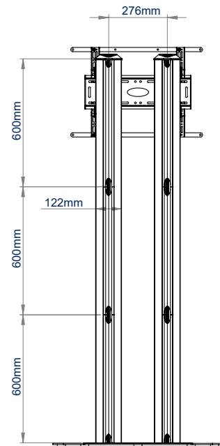
VISTA TRASERA
