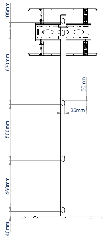
VISTA TRASERA
