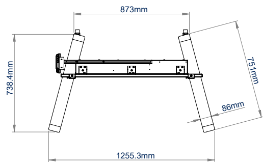
VISTA SUPERIOR
