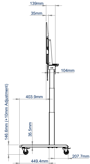
VISTA LATERAL
