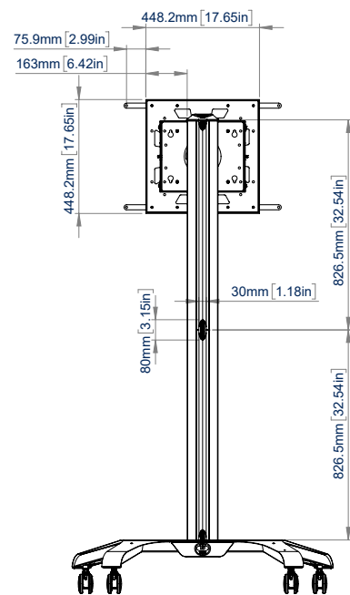
VISTA TRASERA
