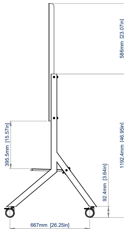
VISTA LATERAL
