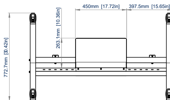
VISTA SUPERIOR
