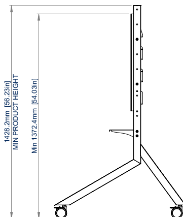
VISTA LATERAL IZQUIERDA ALTURA MÍNIMA
