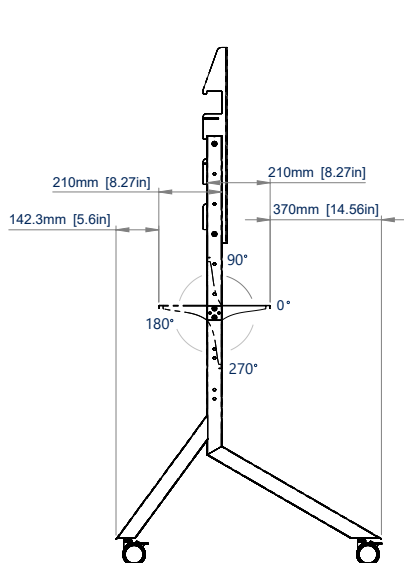
VISTA LATERAL DERECHA ALTURA MÍNIMA
