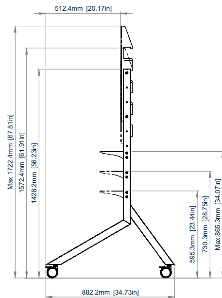
VISTA LATERAL IZQUIERDA ALTURA MÁXIMA
