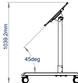
45° INCLINACIÓN
