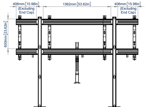
VISTA TRASERA
