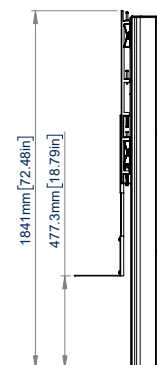
VISTA LATERAL
