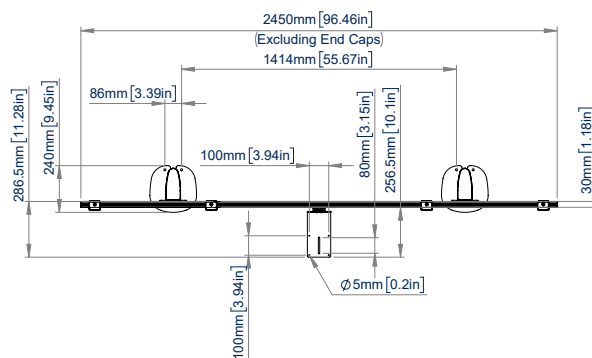
VISTA SUPERIOR
