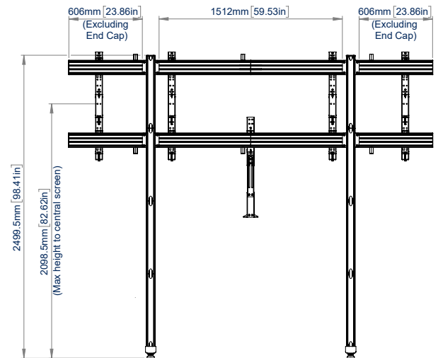
VISTA TRASERA
