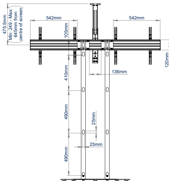
VISTA TRASERA
