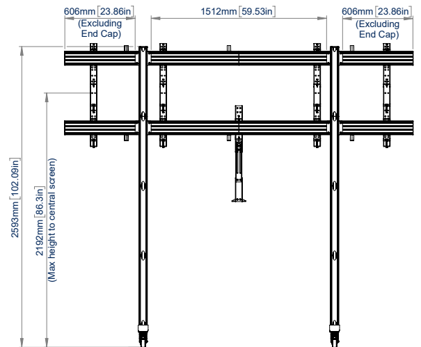
VISTA TRASERA
