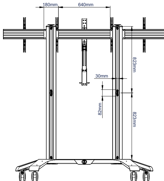
VISTA TRASERA
