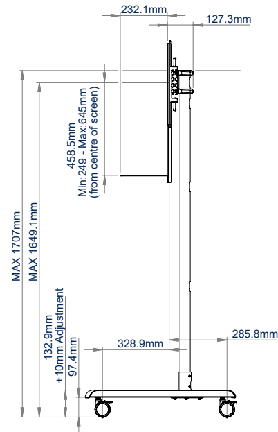
VISTA LATERAL
