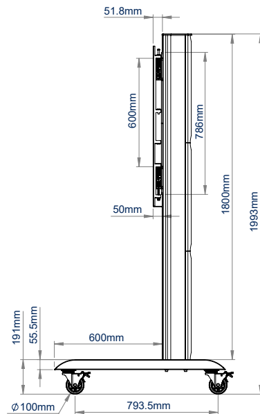
VISTA LATERAL
