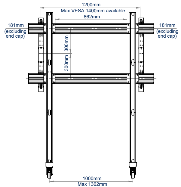
VISTA TRASERA
