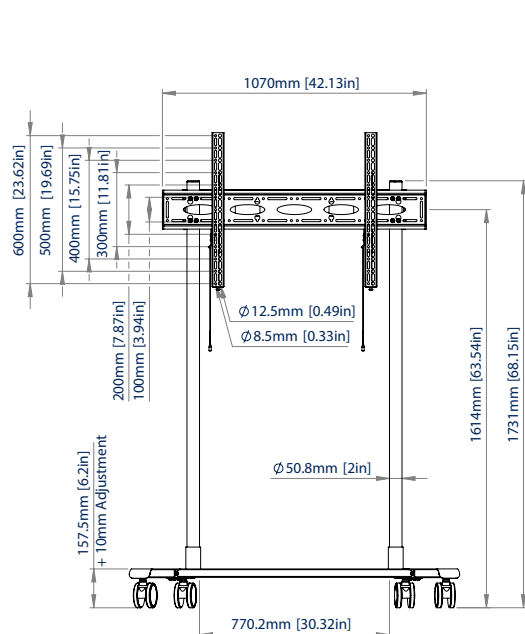
VISTA FRONTAL CON CASTORS
