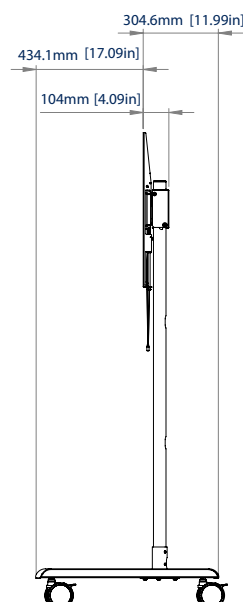
VISTA LATERAL CON CASTORS
