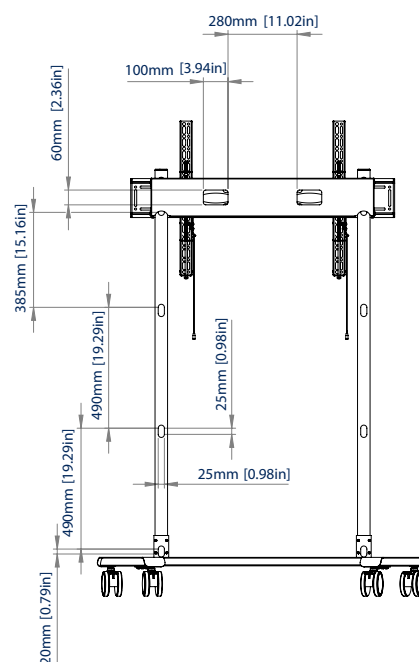
VISTA TRASERA CON CASTORS
