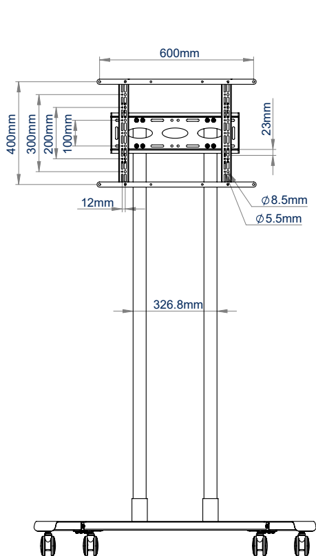
VISTA FRONTAL CON RUEDAS
