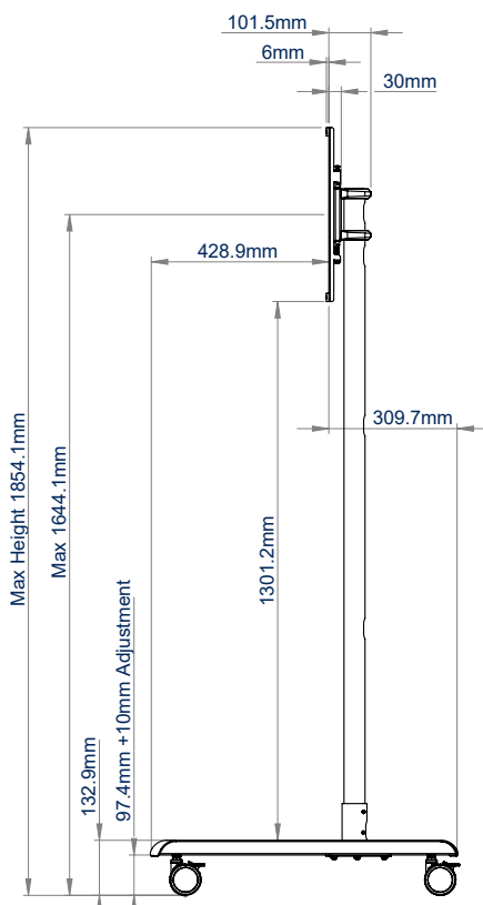
VISTA LATERAL CON RUEDAS
