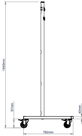
VISTA LATERAL CON CASTORS
