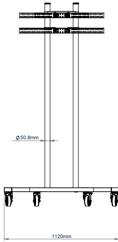
VISTA FRONTAL CON CASTORS
