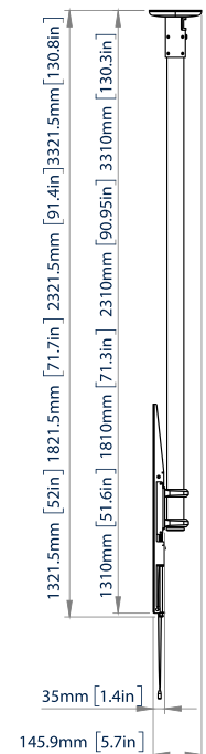
VISTA LATERAL
