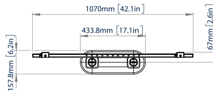
PLACA DE TECHO VISTA SUPERIOR
