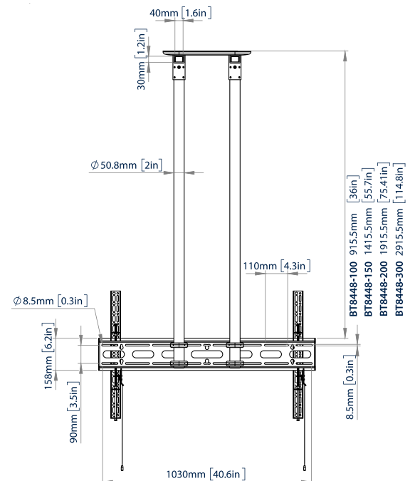
VISTA TRASERA
