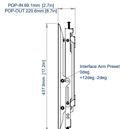
VISTA LATERAL RETIRADO
