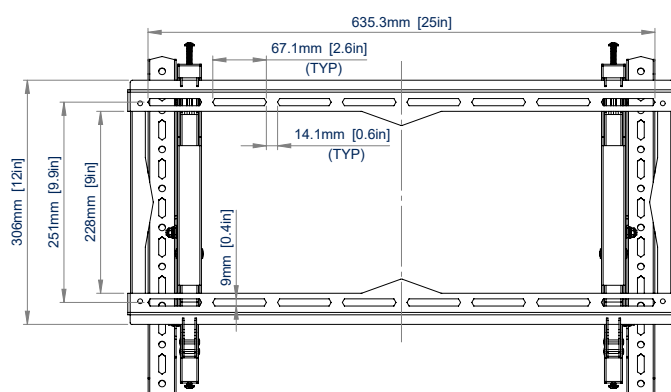
VISTA TRASERA
