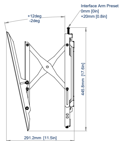
VISTA LATERAL AMPLIADO
