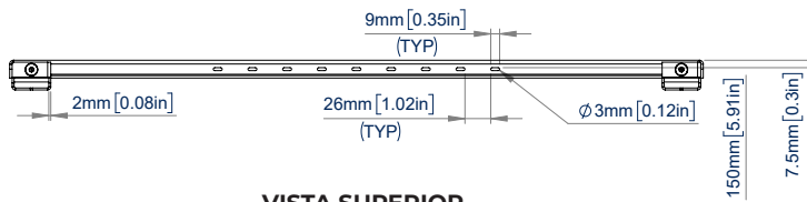
VISTA SUPERIOR
