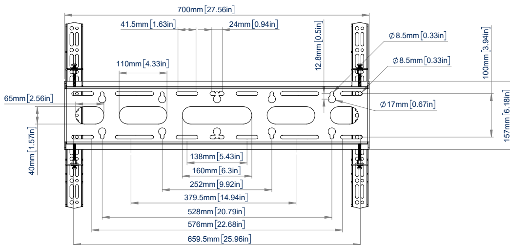
VISTA TRASERA
