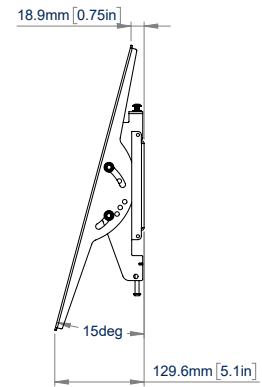
VISTA LATERAL MÍNIMO INCLINACIÓN
