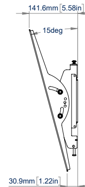
VISTA LATERAL INCLINACIÓN MÁXIMA
