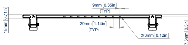
VISTA SUPERIOR
