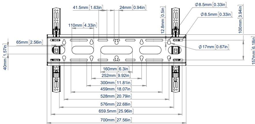
VISTA TRASERA
