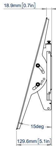
VISTA LATERAL INCLINACIÓN MÁXIMA
