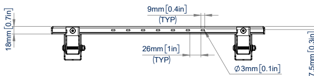
VISTA SUPERIOR
