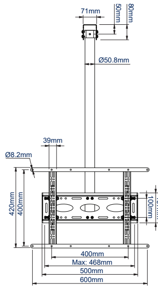
VISTA FRONTAL CON BRAZOS ADAPTADORES
