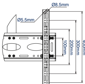
BRAZO DE INTERFAZ VISTA DE CERCA
