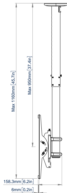
VISTA LATERAL EXTENSIÓN MÁXIMA
