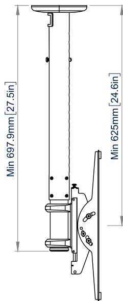
VISTA LATERAL EXTENSIÓN MÍNIMA
