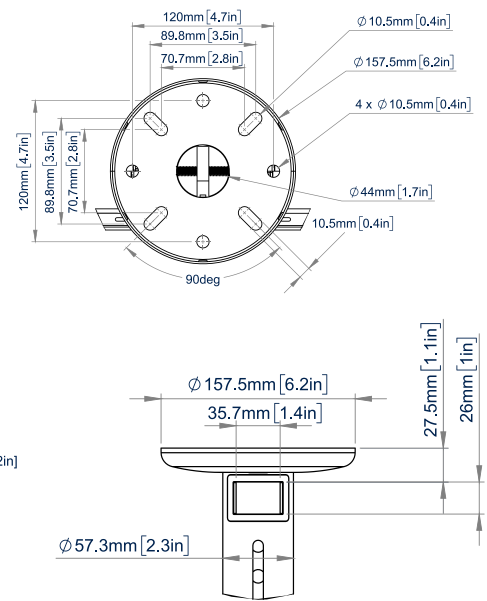
VISTA SUPERIOR
