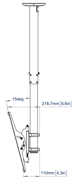
VISTA LATERAL CON INCLINACIÓN
