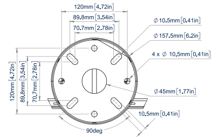
SOPORTE DE TECHO PRIMER PLANO
