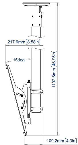
VISTA LATERAL INCLINAR HACIA ABAJO
