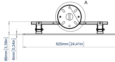
SOPORTE DE TECHO VISTA DESDE ARRIBA
