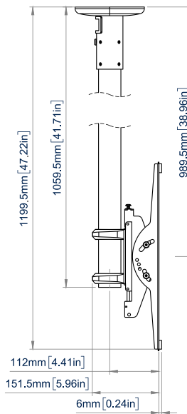
VISTA LATERAL SIN INCLINACIÓN
