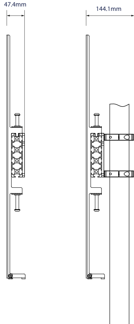
PARA MONTAJE EN PARED A LO LARGO DE UN RIEL*
