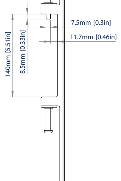
VISTA LATERAL
