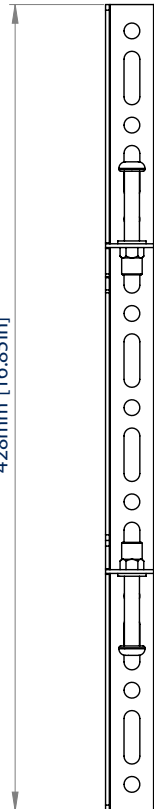
VISTA TRASERA
