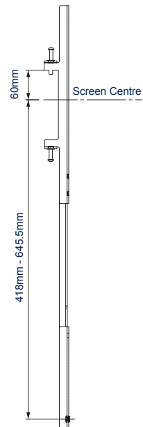
VISTA LATERAL CON BARRA DE EXTENSIÓN - POR DEBAJO DEL RIEL
