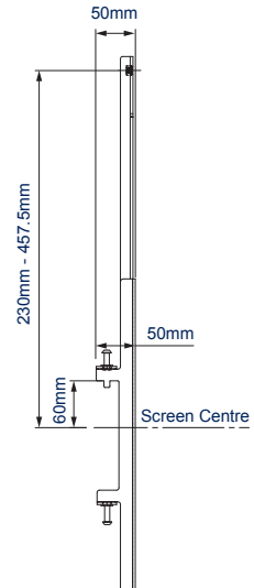
VISTA LATERAL POR ENCIMA DEL RIEL
