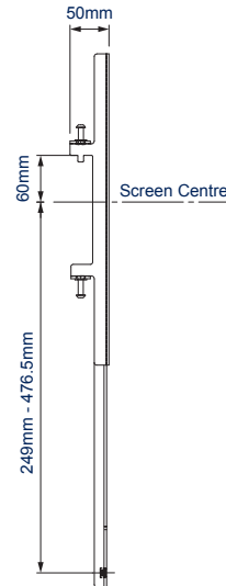
VISTA LATERAL POR DEBAJO DEL RIEL
