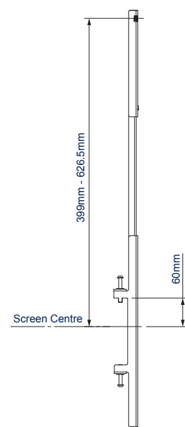
VISTA LATERAL CON BARRA DE EXTENSIÓN - POR ENCIMA DEL RIEL
