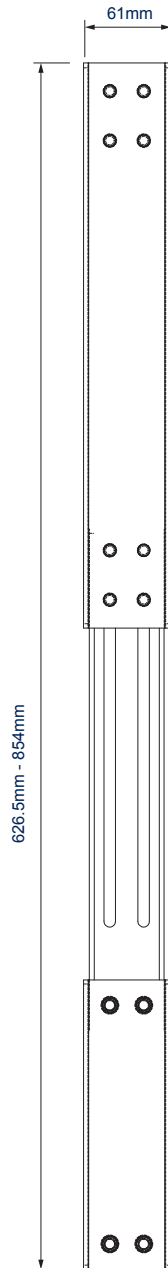
VISTA FRONTAL CON BARRA DE EXTENSIÓN
