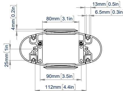
VISTA DESDE ABAJO
