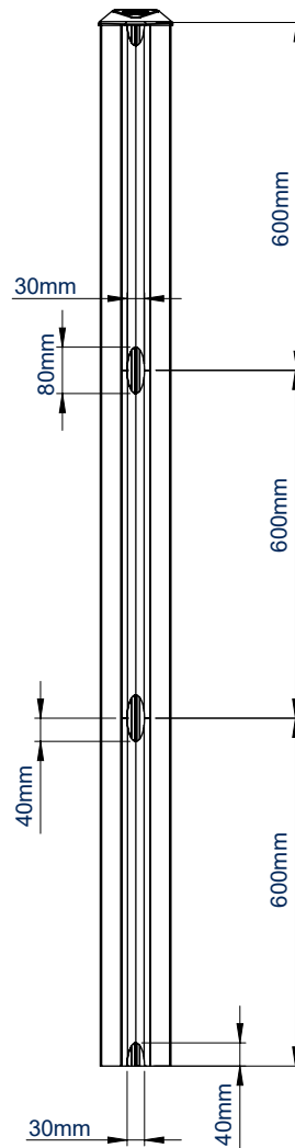
VISTA TRASERA
