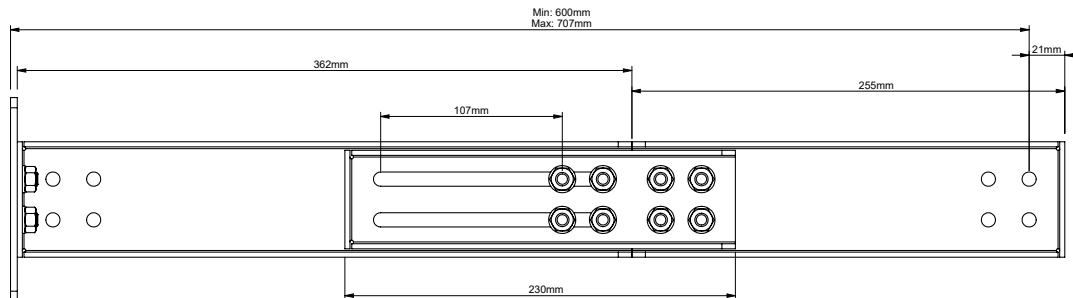
VISTA LATERAL - PLACA DE CONEXIÓN CON UNA PLACA DE EXTENSIÓN LARGA
