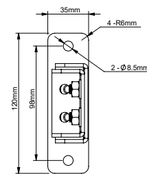
VISTA FRONTAL - PLACA DE PARED
