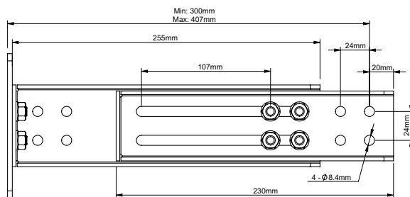
VISTA LATERAL - PLACA DE CONEXIÓN CON UNA PLACA DE EXTENSIÓN CORTA
