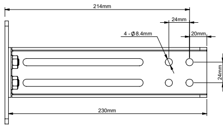
VISTA LATERAL - PLACA DE CONEXIÓN
