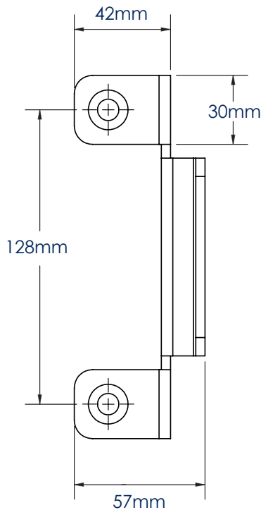
VISTA LATERAL
