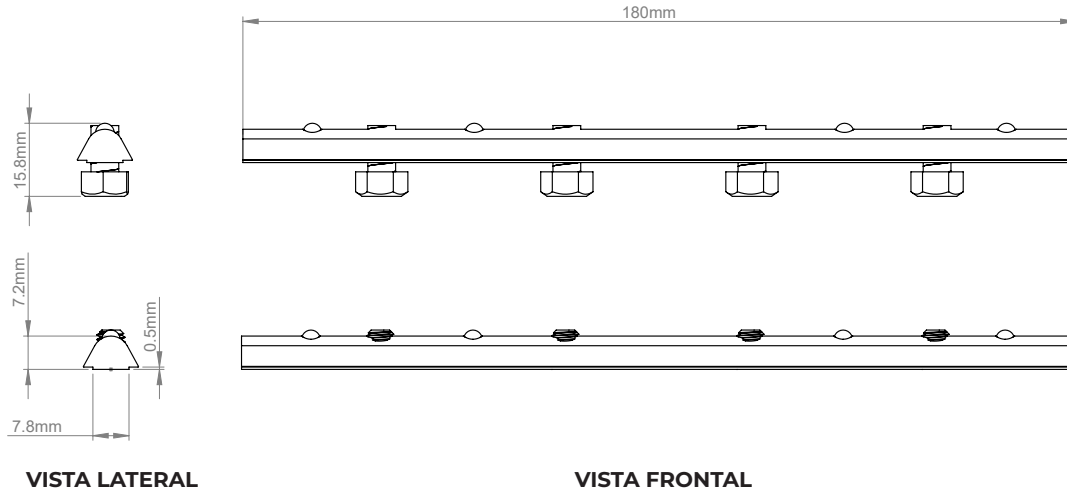
VISTA LATERAL
