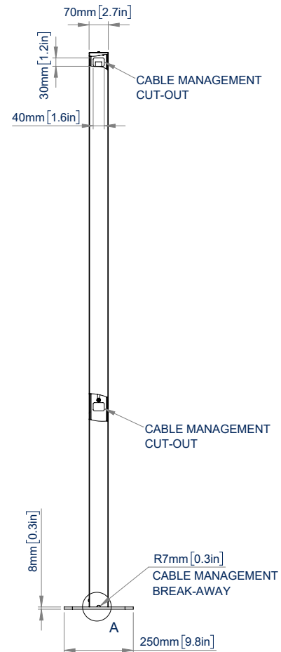
VISTA LATERAL
