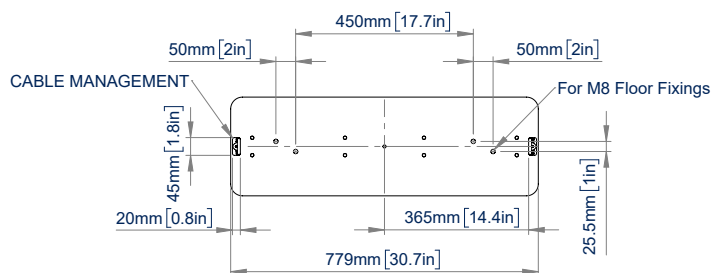
VISTA DESDE ARRIBA
