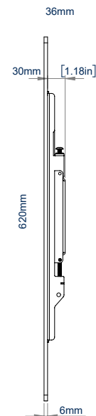
VISTA LATERAL
