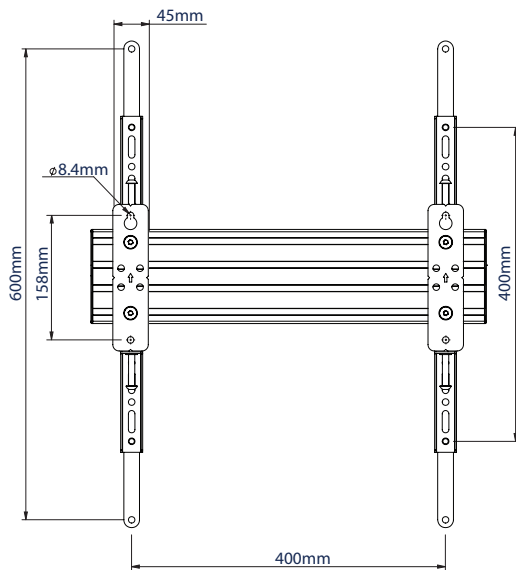
VISTA TRASERA
